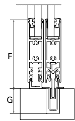
Doorlopende ondergeleiding met plintprofiel
