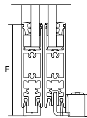
Vastpuntgeleiding met plintprofiel
