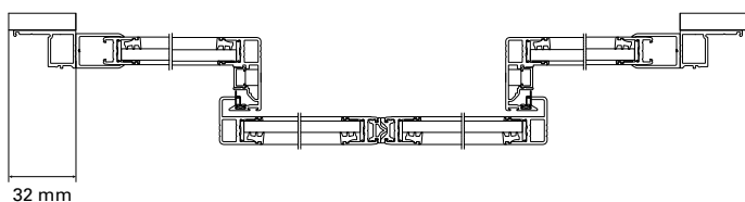
Aan de latei bevestigd
