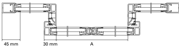
Aan de muur bevestigd
