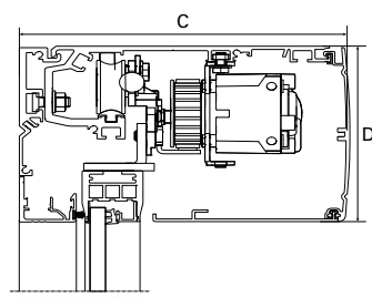
Zonder zijpaneel, met montageprofielen
