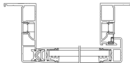
Aan de latei bevestigd
