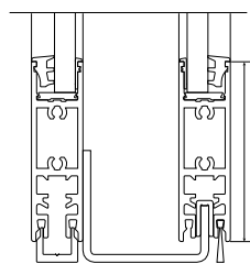
Vastpuntgeleiding
