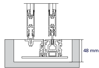
Doorlopende ondergeleiding
